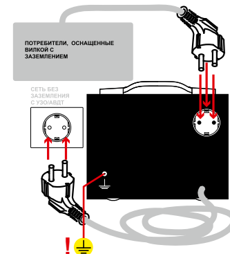
Схема подключения стабилизатора в сеть без заземляющего провода, с УЗО
